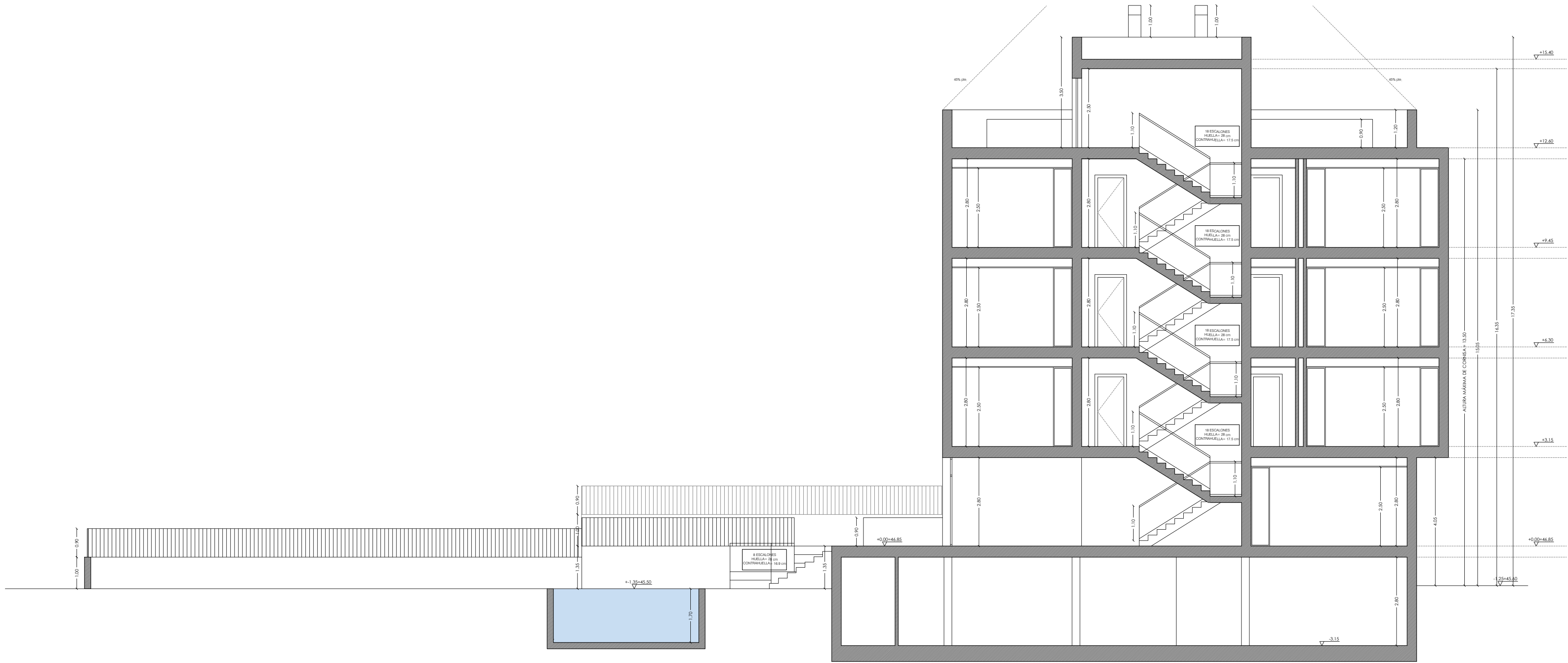
SECCIÓN TRANSVERSAL 1
