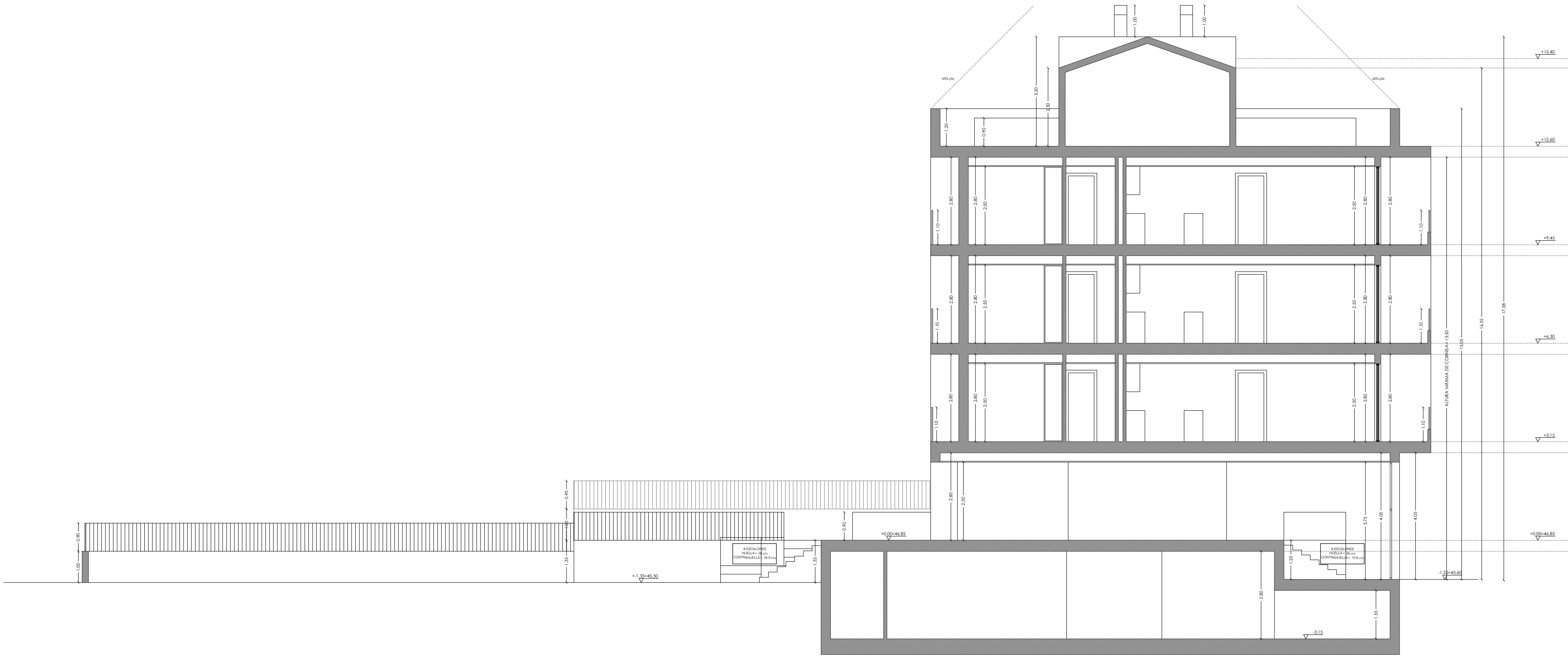
SECCIÓN TRANSVERSAL 2
